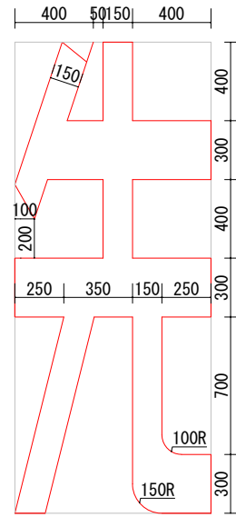
面積 1.152㎡ Le=7.68m LP=9.2m
