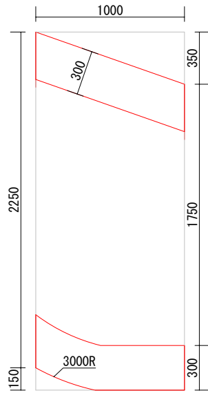
面積 0.626㎡ Le=4.17m LP=5.0m
