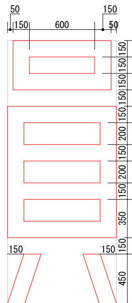
面積 1.078㎡ Le=7.18m LP=8.6m
