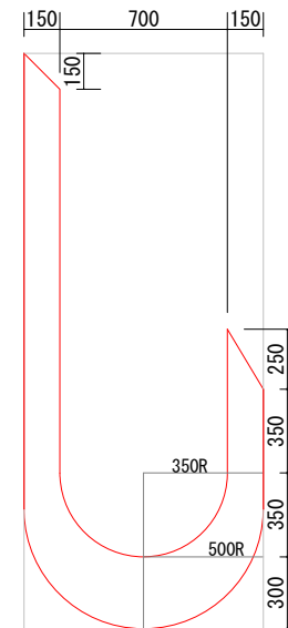
面積 0.680㎡ Le=4.53m LP=5.4m
